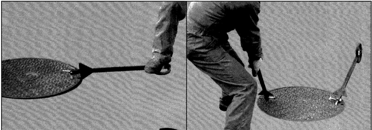
①縁切り
